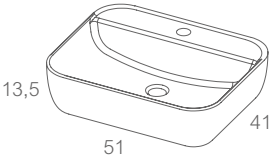
lav. pousar_ HAIA cerâmico
